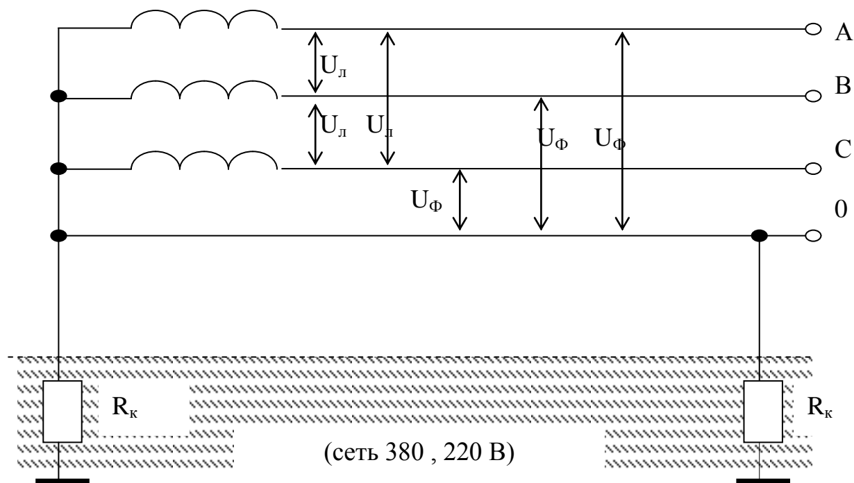
Рис. 2. Схема электрической четырехпроводной
