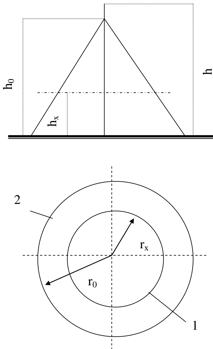
Рис. 3. Зона защиты одиночного стержневого молниеотвода
